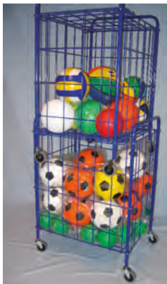
Ballwagen stapelbar dadurch doppelter Stauraum auf gleicher Grundfläche, Stahlkonstruktion, blau lackiert, 4 Lenkrollen für leichten Transport, Maße: (LxBxH) ca. 68 x 53 x 95 cm, Tragkraft: ca. 30 kg
