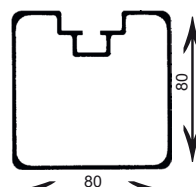
Profilardarstellung
