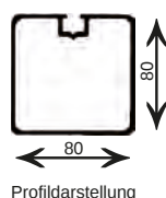
Profildarstellung
