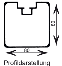
Profilardarstellung
