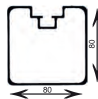
Bodenrahmen
