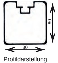
Profilardarstellung
