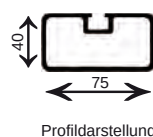
Profilardarstellung
