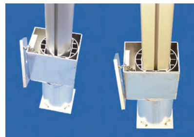
Bodenhülse-Spezial
